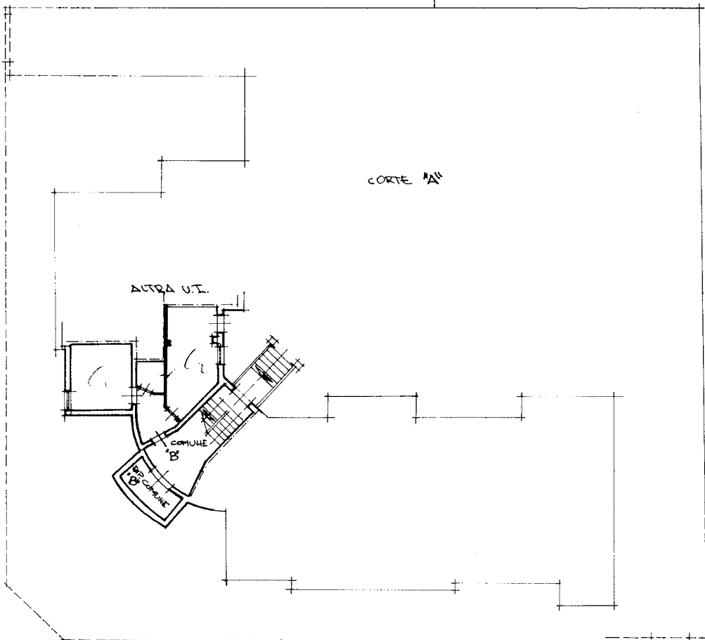
PIANO PRIMO SOTTOSTRADA H=2.55 (SEMINTERRATO)
