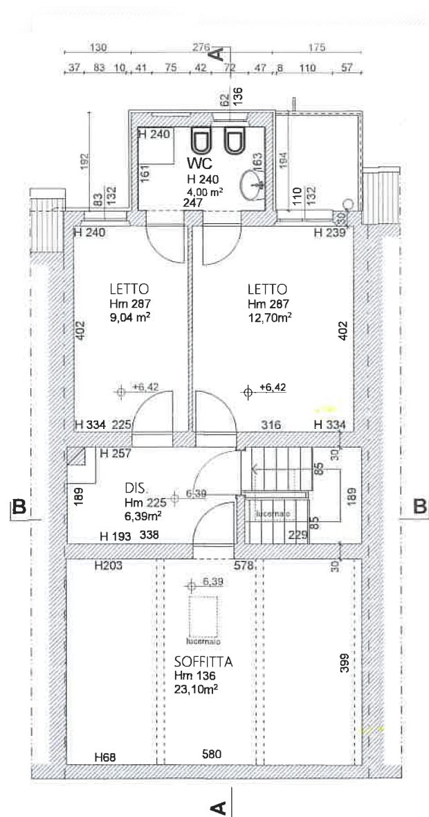
pianta piano secondo sottotetto
