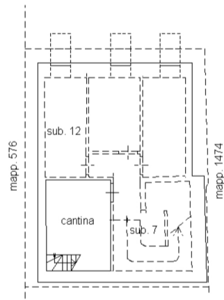
PIANO PRIMO SOTTOSTRADA H=2.10
